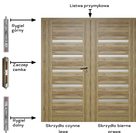
Skrzydła drzwi podwójne z listwą przymykową
