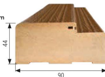
Ościeżnica stała OB-01
