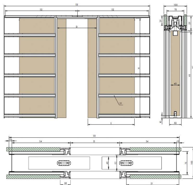
WYMIARY SYSTEMU PODWÓJNEGO (PODANE WYMIARY W MM)
